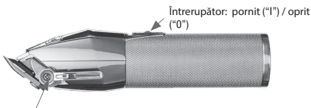
Manetă de reglare a înălțimii de tăiere
